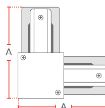
JUNÇÃO L
